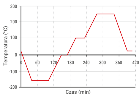
PRZYKŁADOWY PROFIL (obróbka podzerowa i odpuszczanie)
